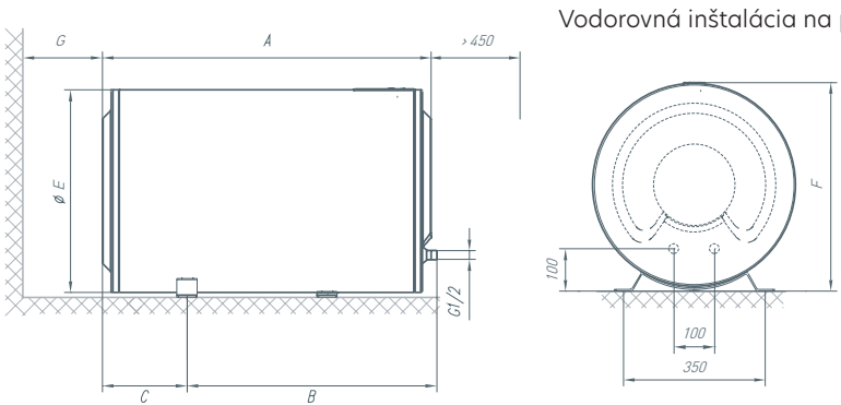
Vodorovná inštalácia na podlahu
