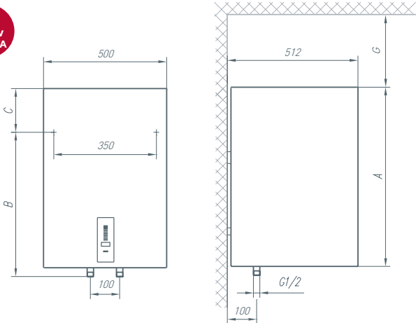
Zvislá inštalácia na stenu
