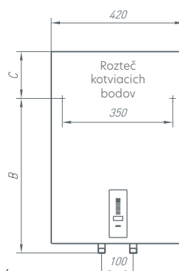
Zvislá inštalácia na stenu
