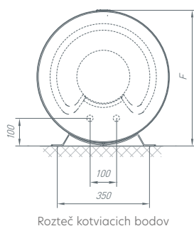
Rozteč kotviacích bodov
